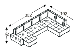
kombinace do tvaru "U" (S1 + R1 + R2L + boční díl B) rozklad pro spaní 140*280 cm
