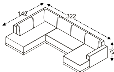
kombinace do tvaru "U" (S1 + R1P + R2L) rozklad pro spaní 140*285 cm
