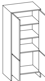
střední skříň 306.046055 š*v'h: 62*137*28 cm
